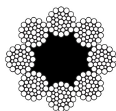
8 x 31 WS FC 1+6+6/6+12
