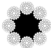
8 x 46 WS FC 1+9+9/9+18
