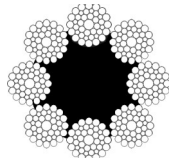
8 x 49 WS FC 1+8+8+8/8+16
