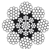
8 x 19 W IWRC 1+6+6/6
