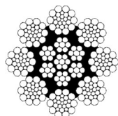
8 x 26 WS IWRC 1+5+5/5+10
