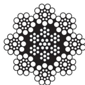
8 x 19 S IWRC 1+9+9
