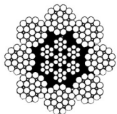
8 x 25 F IWRC 1+6+6F+12
