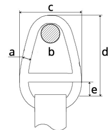
Dimensions des anneaux mâles / Rings dimensions (male type)
