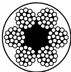
6x19 FC 1+6+12
