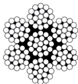
6 x 19 WSC 1+6+12
