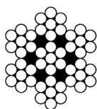
6 x 7 WSC 1+6
