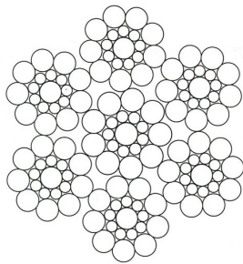
6x19S WSC 1-9-9
