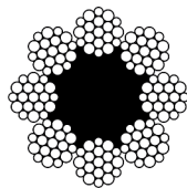
8 x 19 W FC 1+6+6/6
