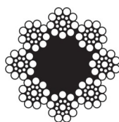
8 x 19 S FC 1+9+9
