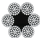
6 x 37 FC 1+6+12+18
