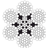
6 x 36 WS IWRC 1+7+7/7+14
