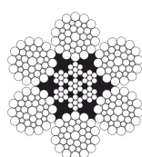
6 x 31 WS IWRC 1+6+6/6+12
