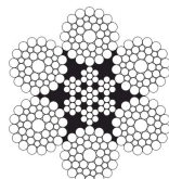
6 x 49 WS IWRC 1+8+8+8/8+16
