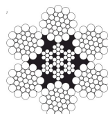
6 x 46 WS IWRC 1+9+9/9+18
