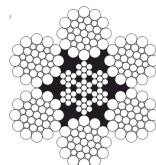
6 x 41 WS IWRC 1+8+8/8+16
