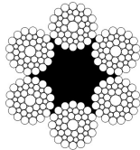
6 x 49 WS AT/FC 1+8+8+8/8+16
