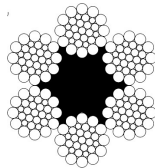
6 x 46 WS AT/FC 1+9+9/9+18
