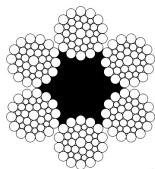
6 x 31 WS AT/FC 1+6+6/6+12
