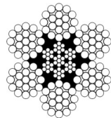
6 x 19 W IWRC 1+6+6/6
