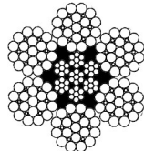
6 x 25 F IWRC 1+6+6F+12
