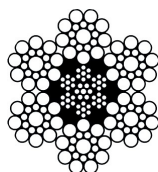
6 x 19 S IWRC 1+9+9
