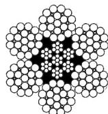
6 x 26 WS IWRC 1+5+5/5+10
