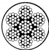
7x19 1+6+12
