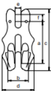
Griffe de raccourcissement à chape avec verrou CL GR100 / Celvis hook CL GR100
