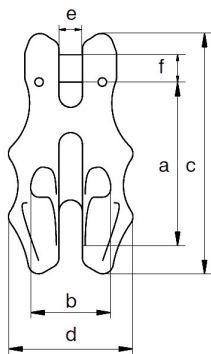
Griffe avec verrou / Clutch with locking
