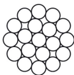
1 x 19 WS 1+6+12
