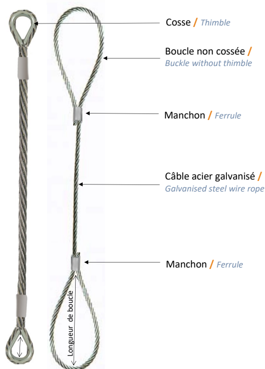
Composition d'une élingue sans terminaison Composition of wire rope without termination
