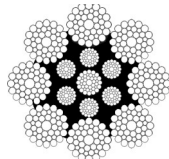
8 x 46 WS IWRC 1+9+9/9+18
