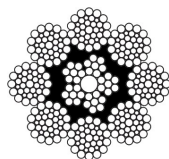
8 x 41 WS IWRC 1+8+8/8+16
