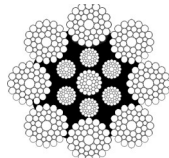
8 x 49 WS IWRC 1+8+8+8/8+16
