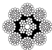
8 x 31 WS IWRC 1+6/6/6+12
