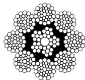
8 x 36 WS IWRC 1+7+7/7+14
